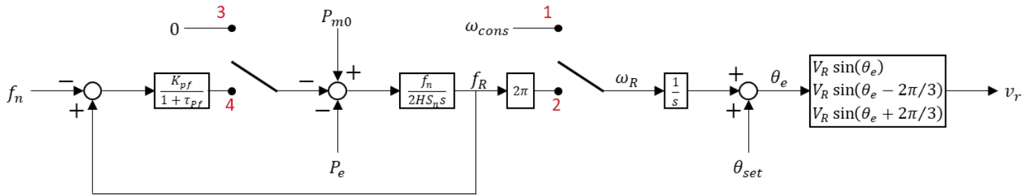
Figure 13 : modèle détaillé de la source de tension V_r
