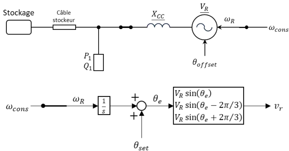
Figure 22 : modèle réseau pour la fiche 6
