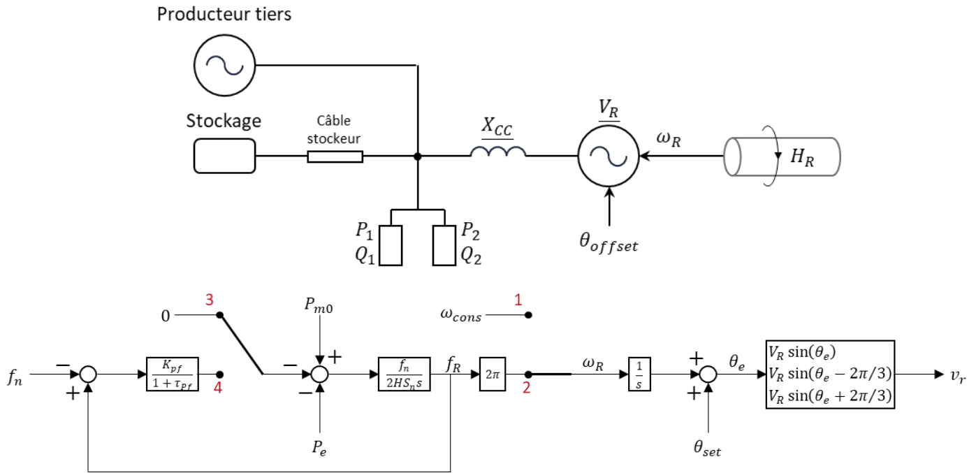
Figure 18 : modèle réseau pour la fiche 4
