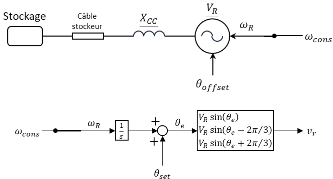
Figure 19 : modèle réseau pour la fiche 5
