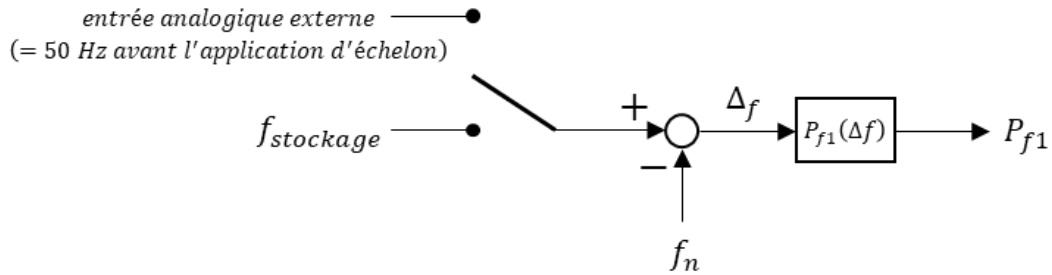
Figure 24 : illustration de la méthode 1 pour s'affranchir des variations de la fréquence du réseau
