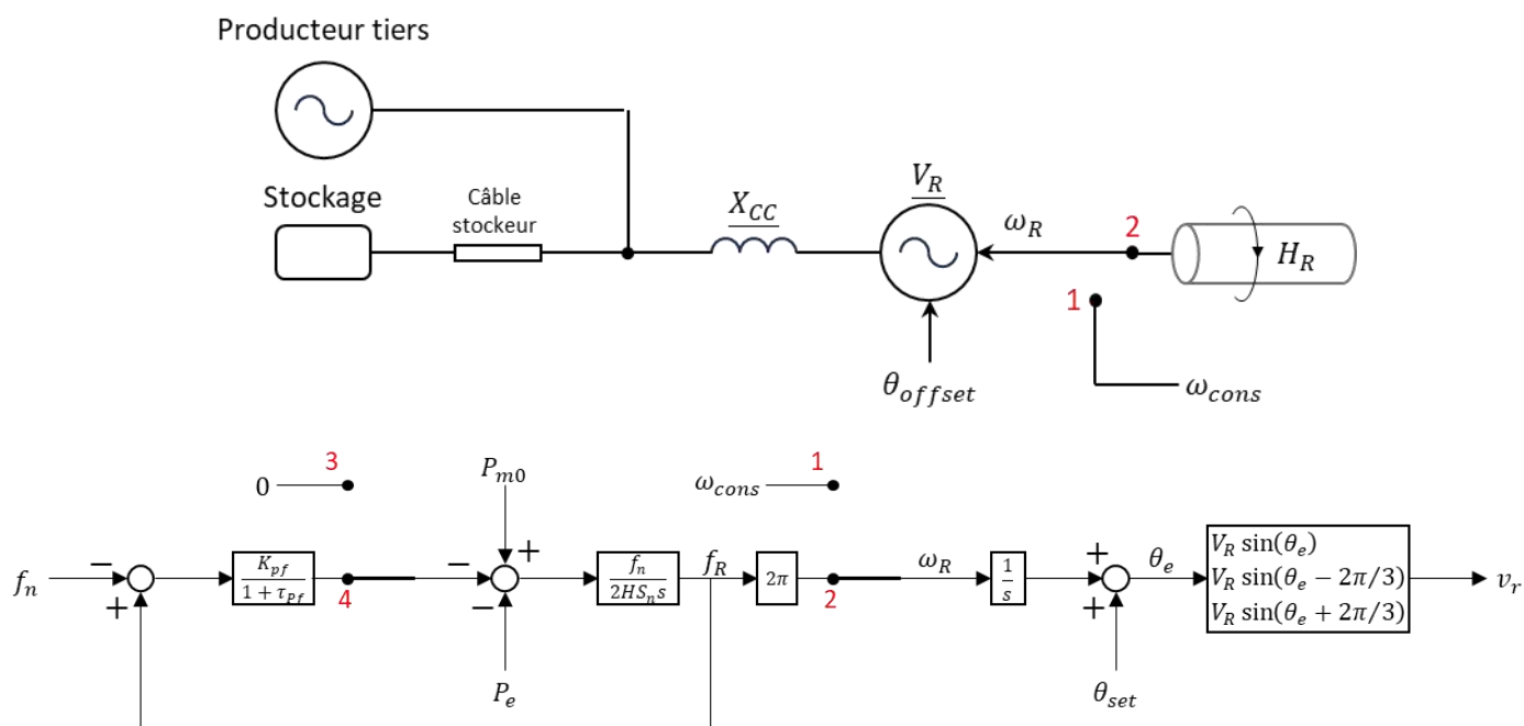
Figure 16 : modèle réseau pour la fiche 2
