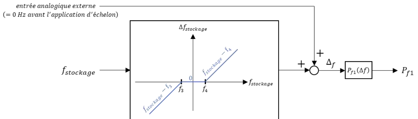
Figure 25 : illustration de la méthode 2 pour s'affranchir des variations de la fréquence du réseau
