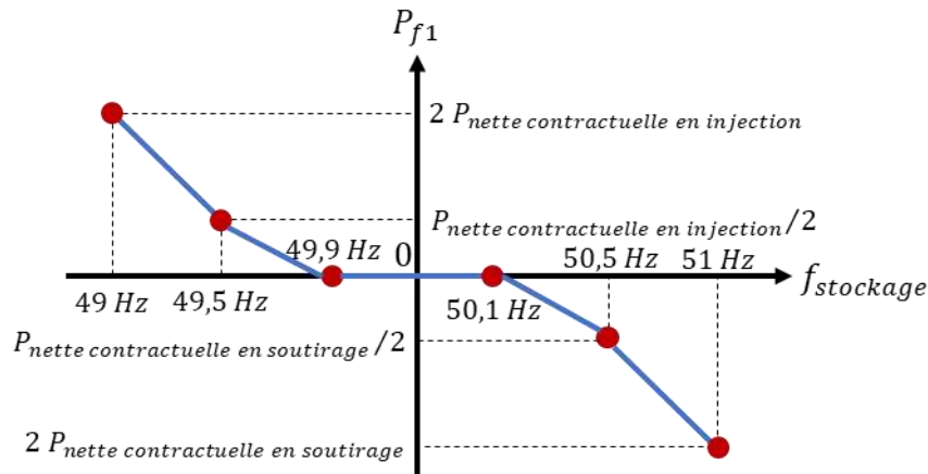
Figure 26 : réglage de la caractéristique de réglage primaire de fréquence
