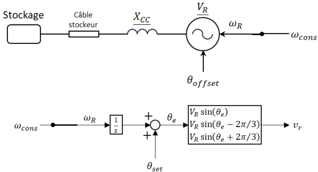
Figure 14 : modèle réseau pour la fiche 1
