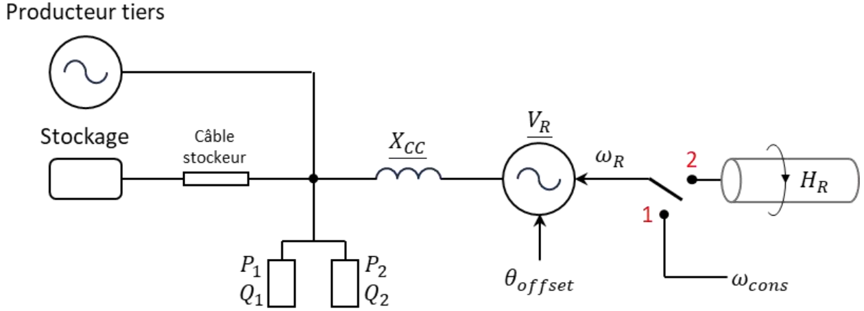
Figure 12 : modèle du réseau
