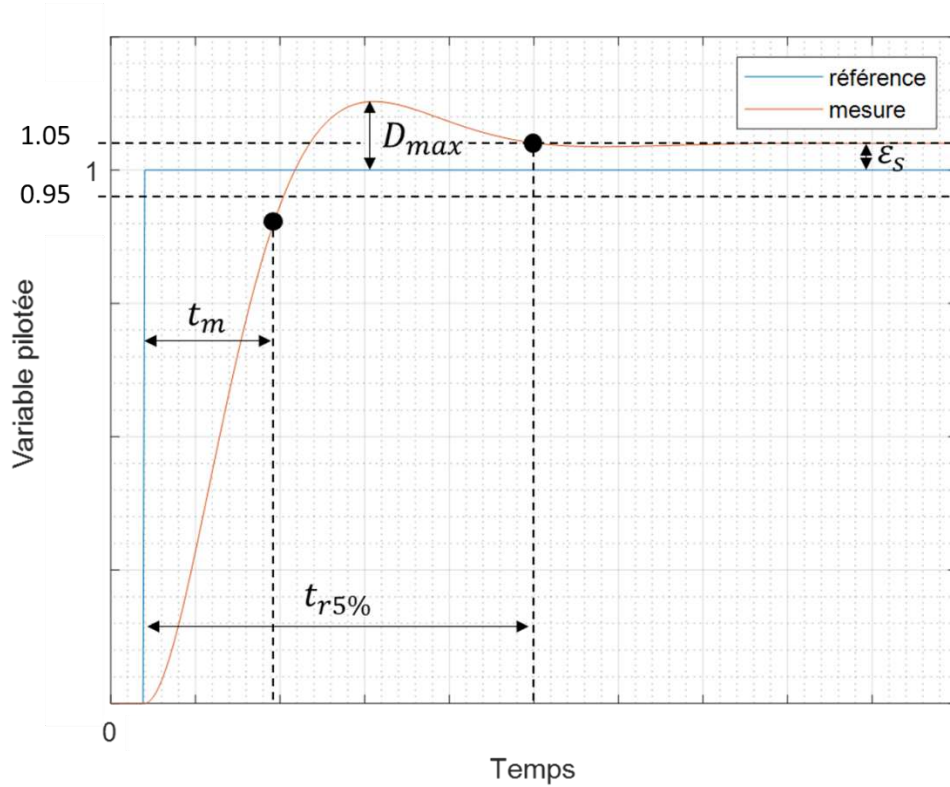
Figure 27 : Définition des performances dynamiques de la réponse à un échelon
