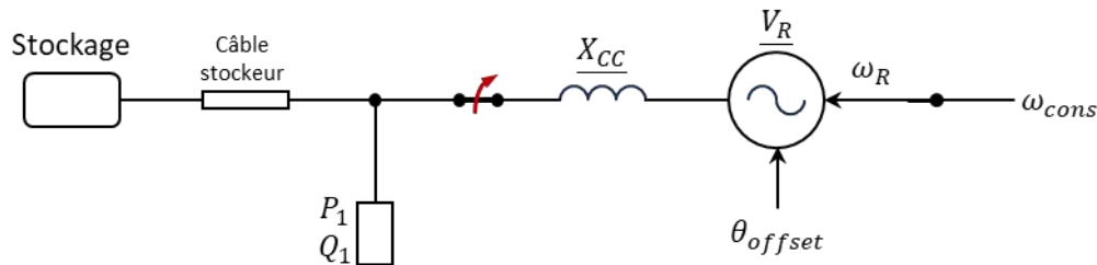
Figure 23 : Ouverture disjoncteur à simuler
