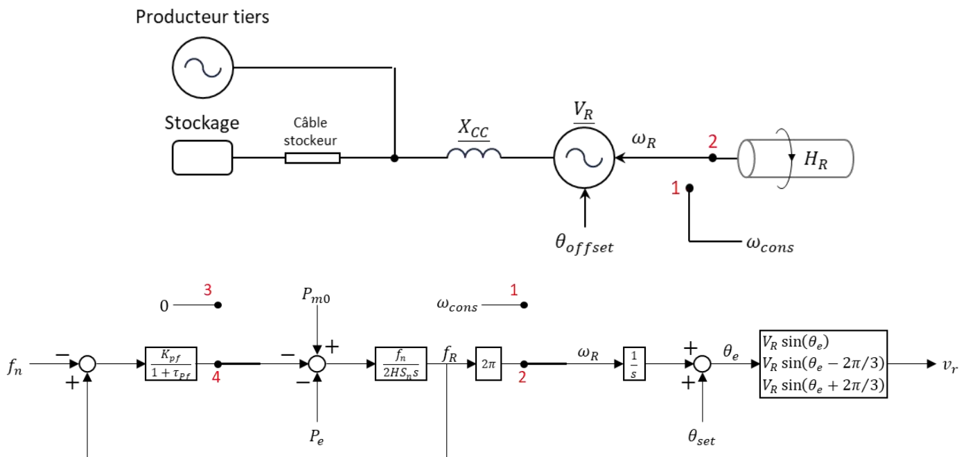
Figure 17 : modèle réseau pour la fiche 3
