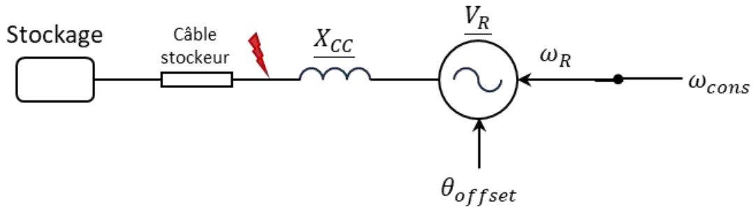
Figure 21 : emplacement du court-circuit triphasé franc à simuler
