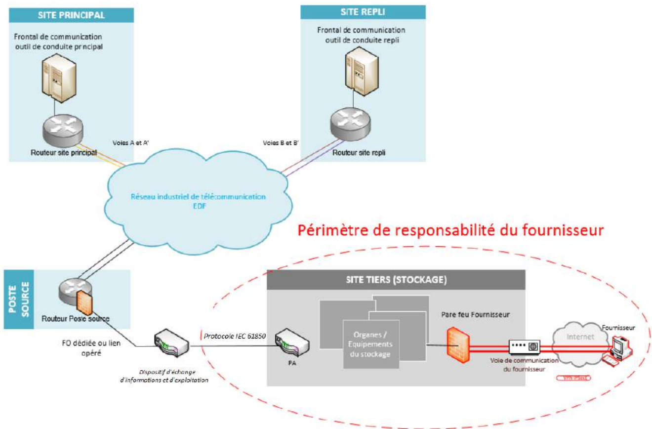
Figure 10 : Schéma de l'architecture de communication
